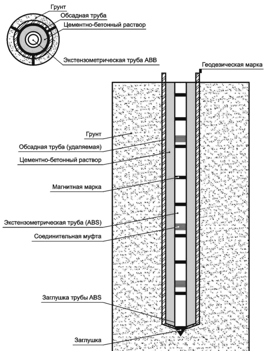
Рисунок Д.2. Схема экстензометрической наблюдательной скважины
