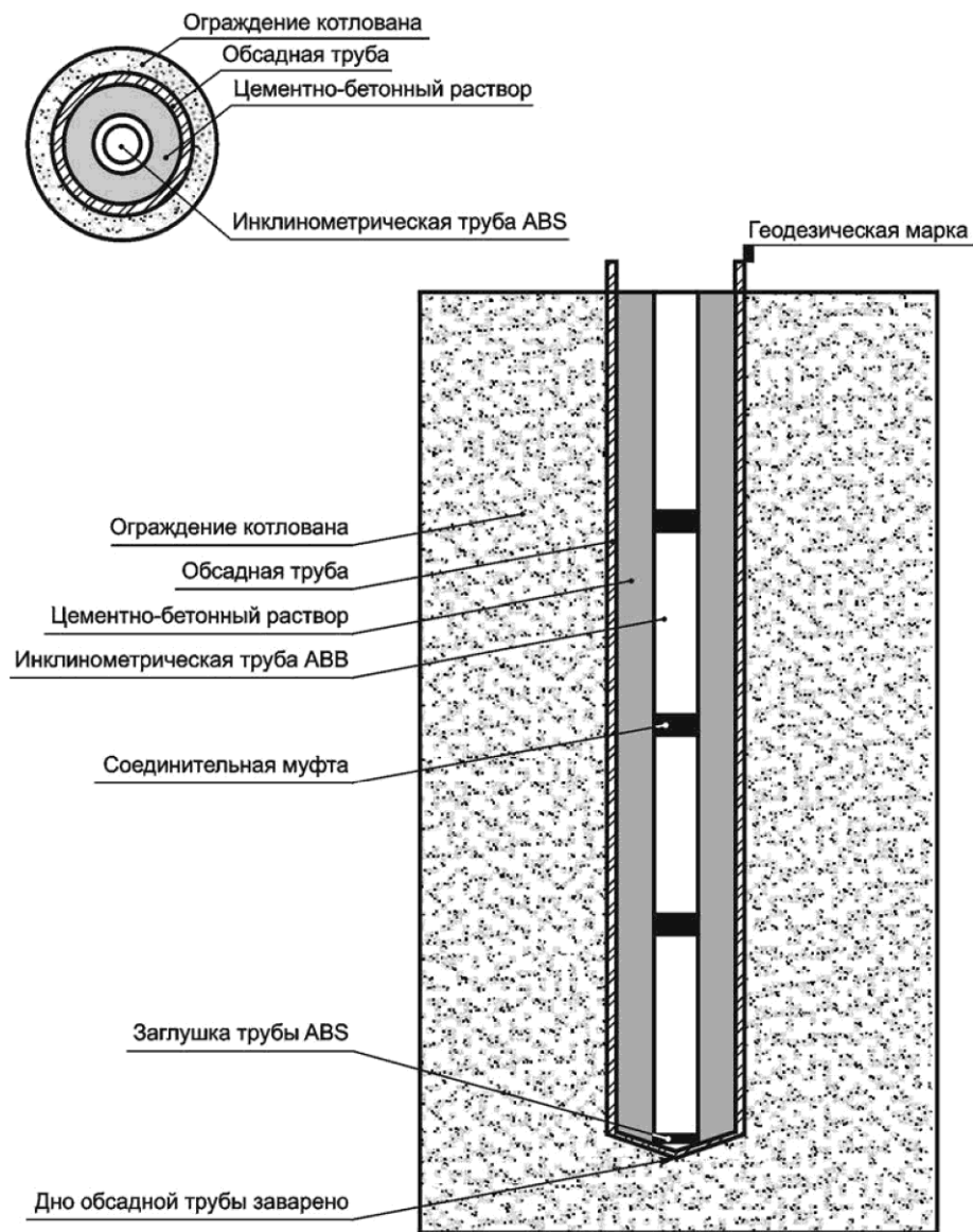
Рисунок Д.1. Схема инклинометрической наблюдательной скважины
